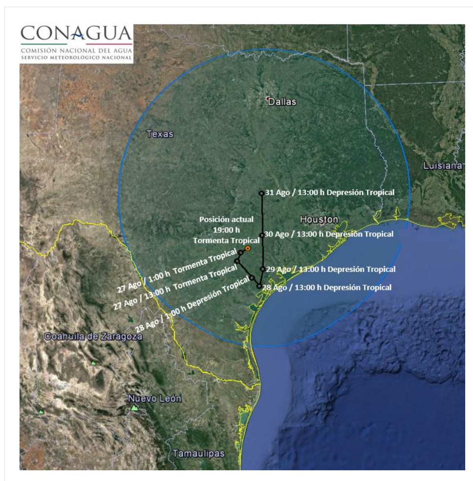
Trayectoria pronóstico de la tormenta tropical "Harvey"
